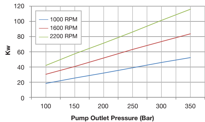
C081 Input Power
